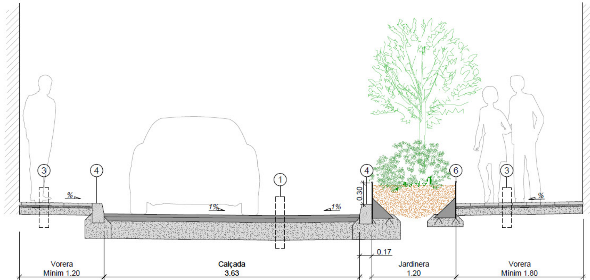
Secció Avinguda Panagall
