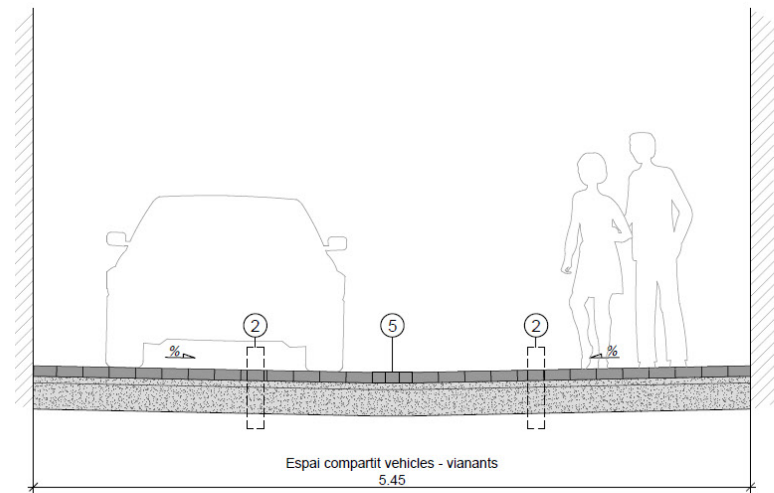
Secció Passatge d'Ausies March
